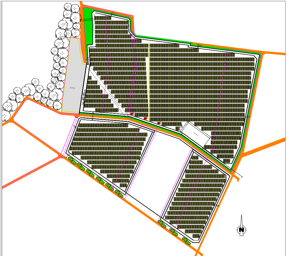
Abb. 4: Vorhaben- und Erschließungsplan (Vorabzug) Quelle: Ranft Projekte 20 GmbH 22.09.2025, unmaßstäblich
